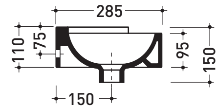
sezione longitudinale / section
