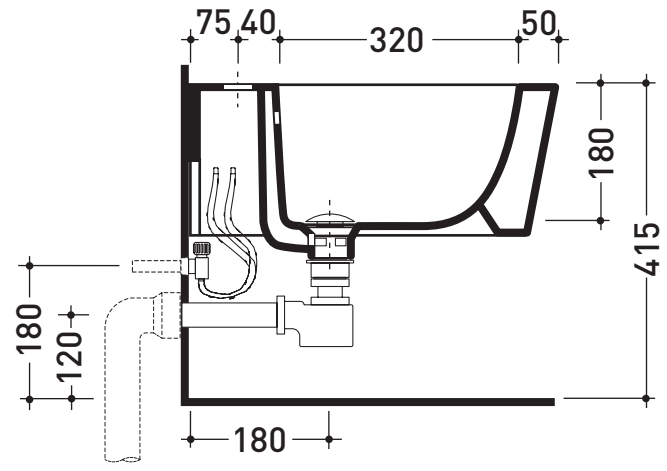
sezione longitudinale / section
