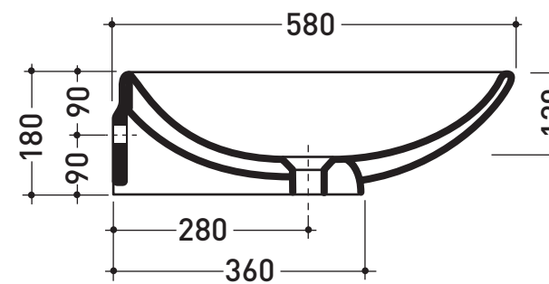
sezione longitudinale / section
