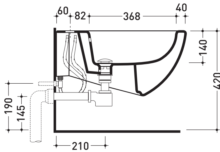
sezione longitudinale / section
