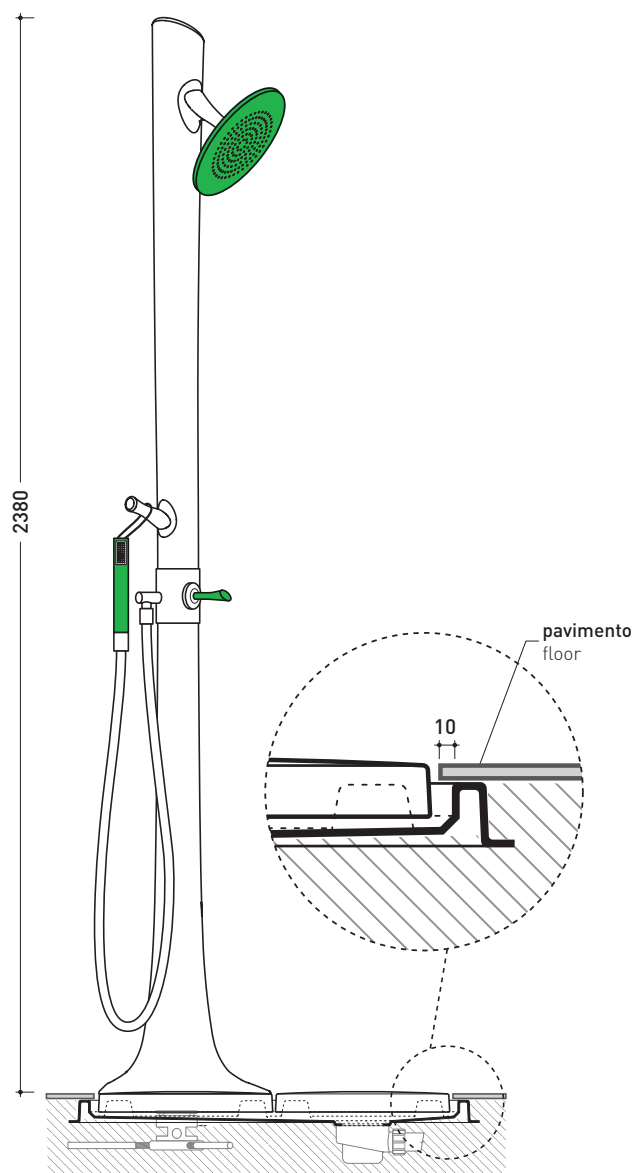
sezione longitudinale / section
