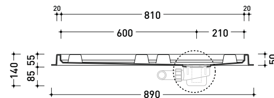
sezione B - B / section B - B
