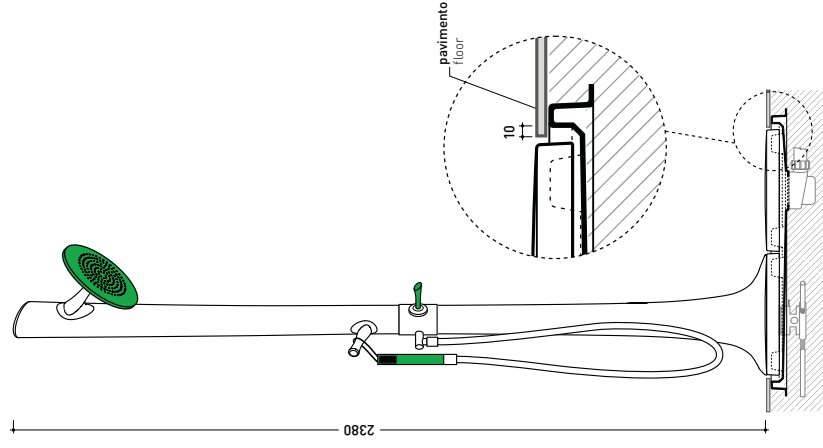
sezione longitudinale / section
