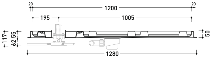
sezione A - A / section A - A
