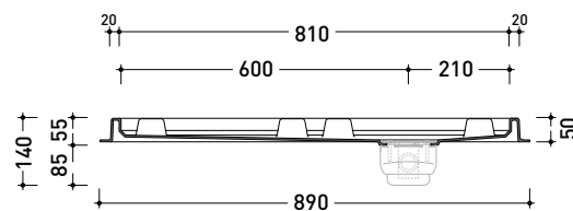
sezione trasversale / section
