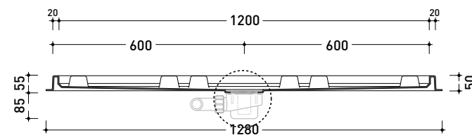
sezione longitudinale / section
