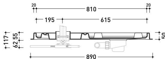
sezione A - A / section A - A
