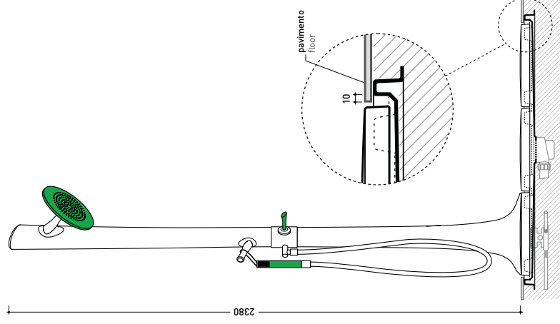
sezione longitudinale / section
