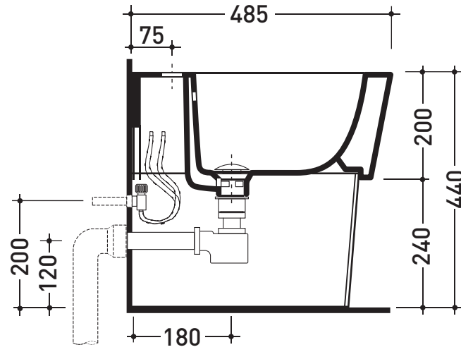
sezione longitudinale / section
