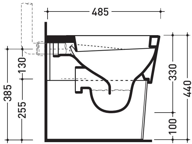
sezione longitudinale / section
