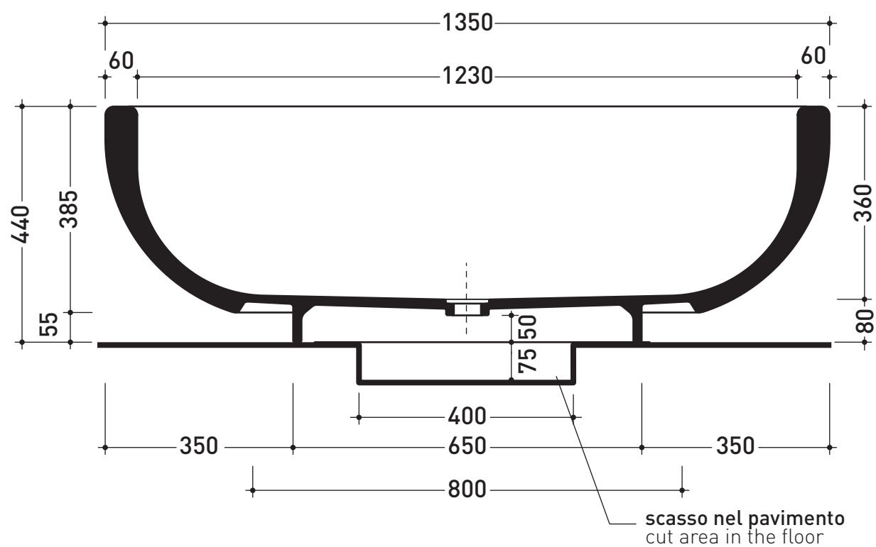
sezione longitudinale / section
