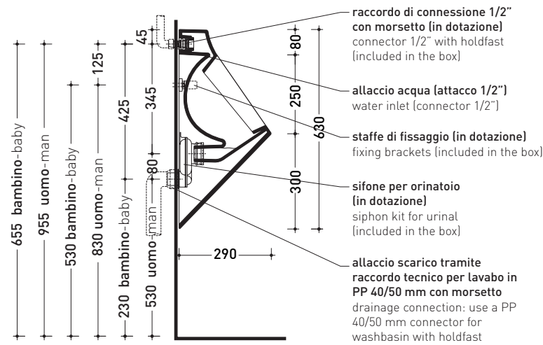
sezione longitudinale / section
