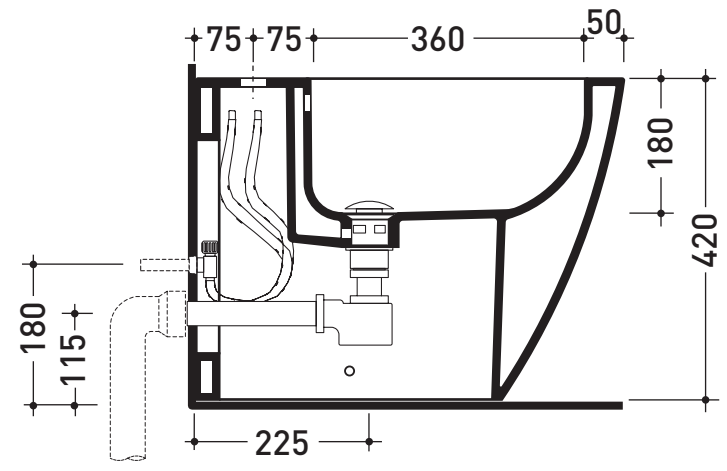
sezione longitudinale / section
