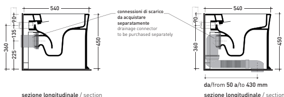
sezione longitudinale / section
