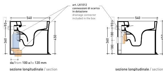
sezione longitudinale / section
