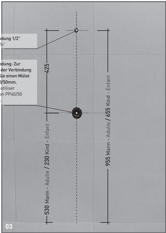
03 Vorbereitung der Installation des Zu- und Abflusses zur Spülung des Urinal. ACHTUNG! Beachten Sie UNBEDINGT die angegebenen Maße! Préparation de l'alimentation en eau et de l'évacuation. Attention, veiller a bien respecter les cotes indiquées.
