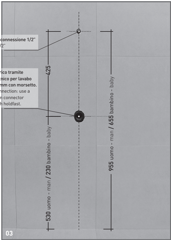
03 Predisposizione dello scarico e dell'adduzione acqua di risciacquo dell'orinatoio. Attenzione: rispettare le misure indicate. Preparation of the drain and water supply for the flushing of the urinal. Attention: make sure to respect the measurements indicated.
