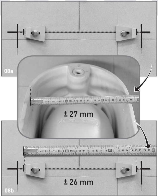
08 Montage der Befestigungslaschen. Schrauben Sie die Laschen an die Wand (8a). Nehmen Sie das Innenmaß des Urinal (±27mm) und überprüfen dann, das der Abstand zwischen den Laschen höchstens 10mm weniger ist als das Innenmaß des Urinal.(±26mm) Ziehen Sie die Schrauben der Befestigungen nach Einrichten fest an. Fixation des équerres: bloquer les deux équerres comme indiqué dans la photo (08a). Mesurez l'intérieur de l'installation sanitaire (± 27 mm) et vérifiez ensuite que la distance entre les équerres soit au moins 10mm (± 26 mm) de moins que la mesure. fixer solidement les équerres dans la position correcte.
