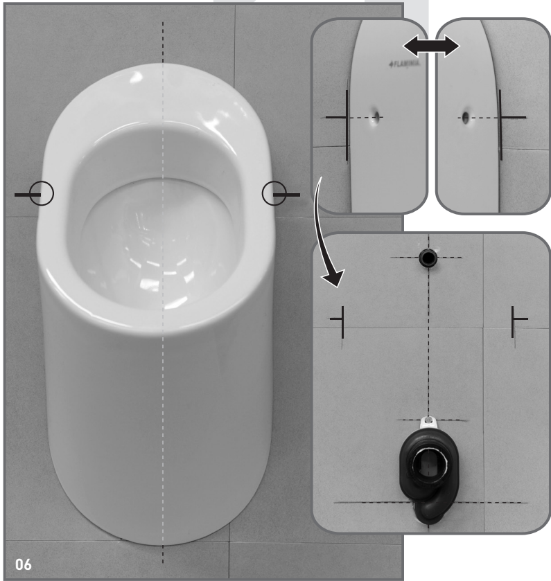
06 Vorereitung zur Installation des Urinal an der Wand. Zeichnen Sie die Außenposition der Befestigungslaschen an der Wand an, nachdem Sie den Sifon und Zulaufgummiverbinder mit Gleitmittel eingestrichen haben. Préparation pour fixer l'urinoir au mur: Monter le sanitaire au mur après avoir lubrifié les parties en caoutchouc. Marquer sur le mur l'emplacement des trous de fixation.
