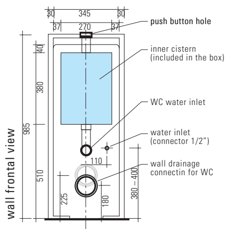
Niagara 39 Art. TR39 Spülkastensystem zu bodenstehendem WC LINK
