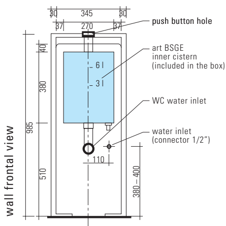
Niagara 38 Art. TR38 Spülkastensystem zu bodenstehendem WC LINK
