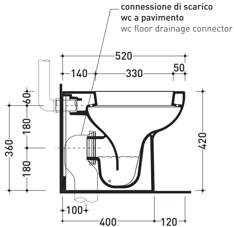
sezione longitudinale / section
