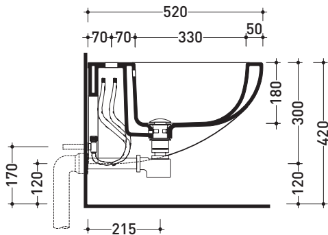
sezione longitudinale / section
