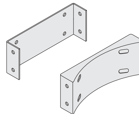
staffa di fissaggio fixing bracket
