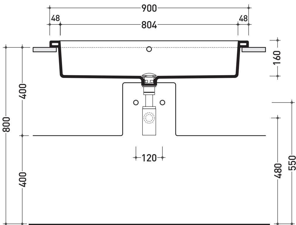
sezione trasversale / section
