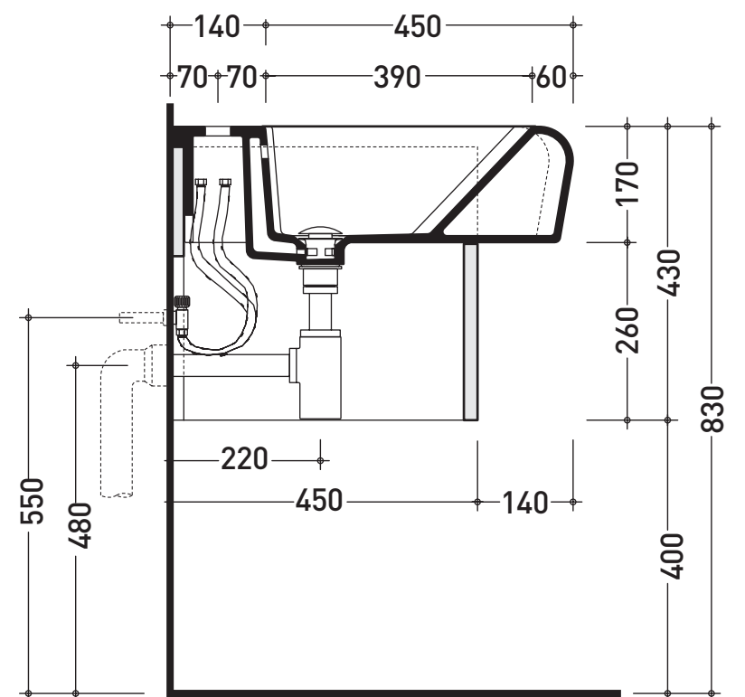
sezione longitudinale / section
